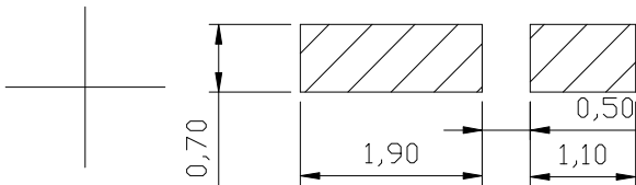
焊盘尺寸
