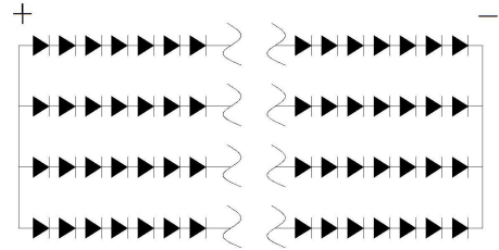
100 串 4 并
