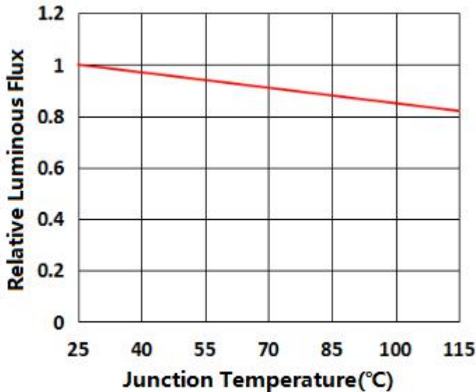
亮度与温度关系曲线图
