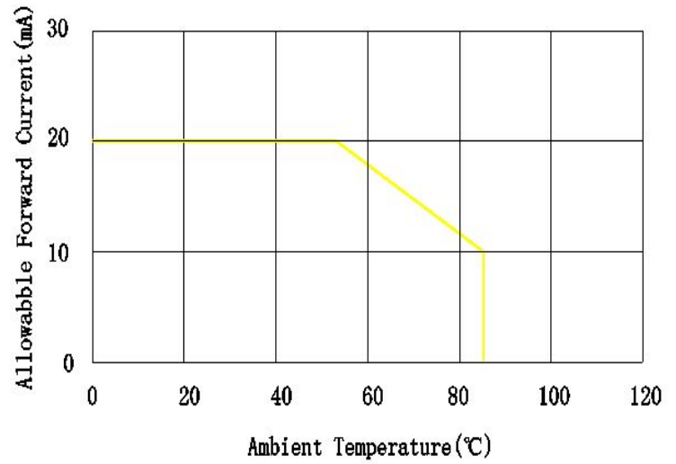
电流与环境温度关系曲线图 Forward Current VS Ambient
