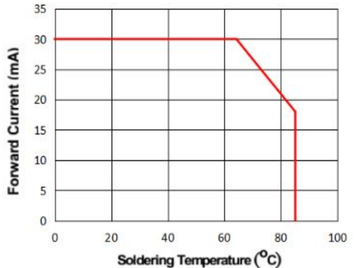
电流与温度关系曲线图
