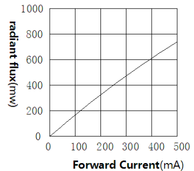
正向电流与辐射功率关系曲线图 Forward Current VS radiant flux
