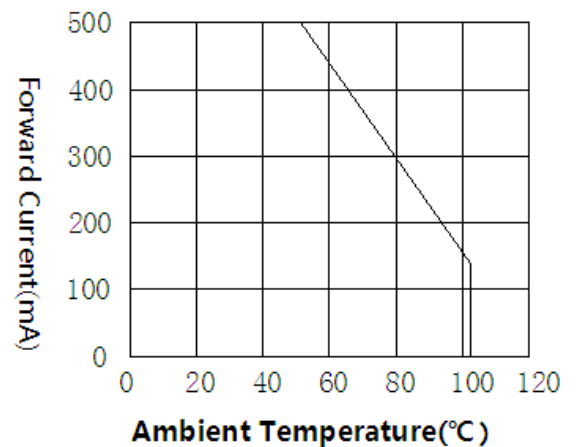
电流与环境温度关系曲线图 Forward Current VS Ambient Temperature
