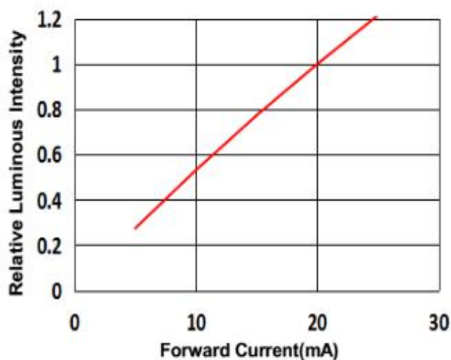
亮度与电流关系曲线图
