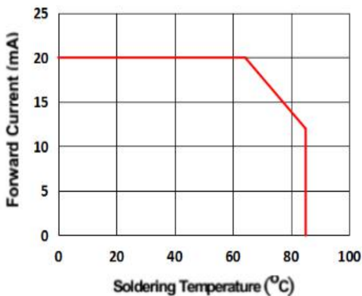
电流与温度关系曲线图
